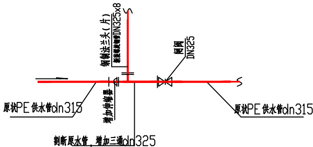
主要节点详图
